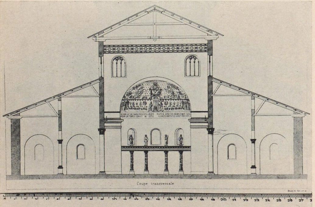
b) P. Letarouilly und Simil, Querschnitt von St. Peter
