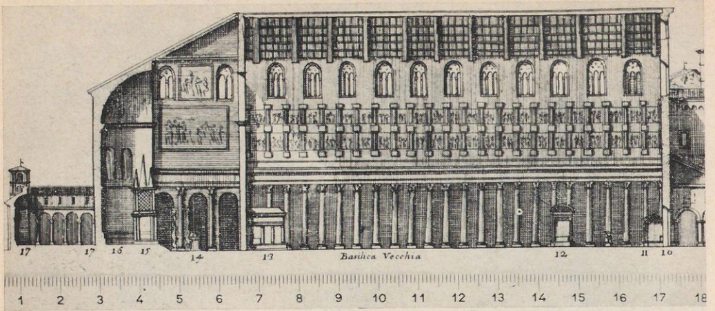
a) C. Fontana, Längsschnitt von St. Peter
