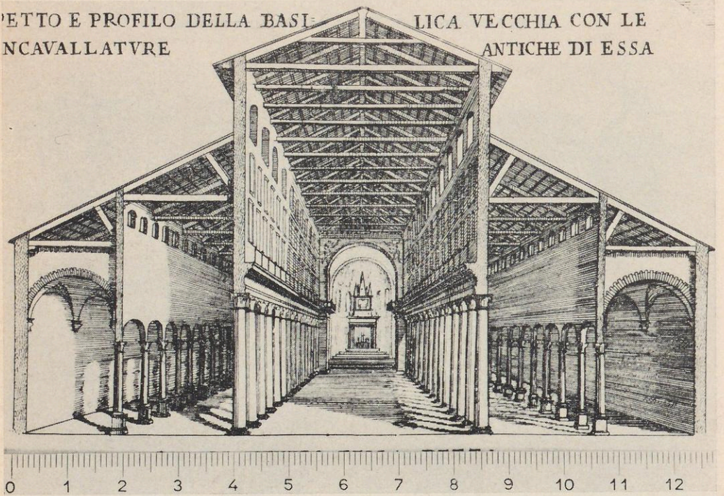
b) C. Fontana, Rekonstruktion der Innenansicht
