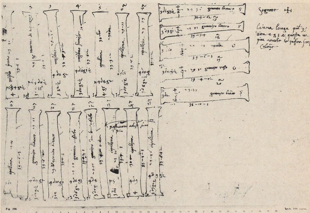
b) B. Peruzzi, Schäfte der linken Mittelschiffskolonnade von Alt-St.-Peter
