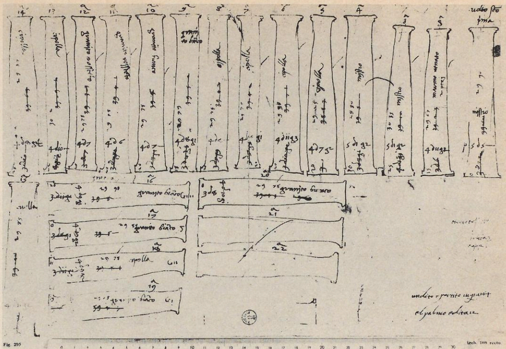
a) B. Peruzzi, Schäfte der rechten Mittelschiffskolonnade von Alt-St.-Peter
