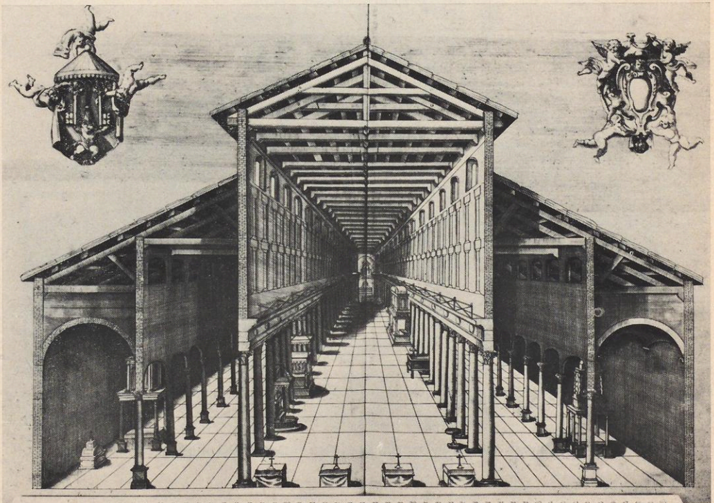
b) M. Ferrabosco, Rekonstruktion der Innenansicht
